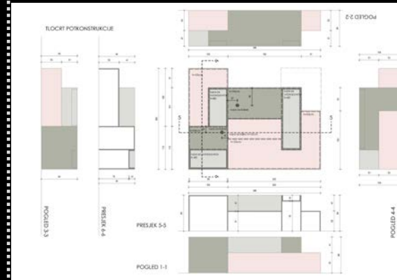
6. Glavni/izvedbeni projekt
